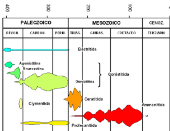
[Figura 52] (sopra) - Distribuzione stratigrafica dei principali gruppi tassonomici degli Ammonoidea - da Wikipedia
