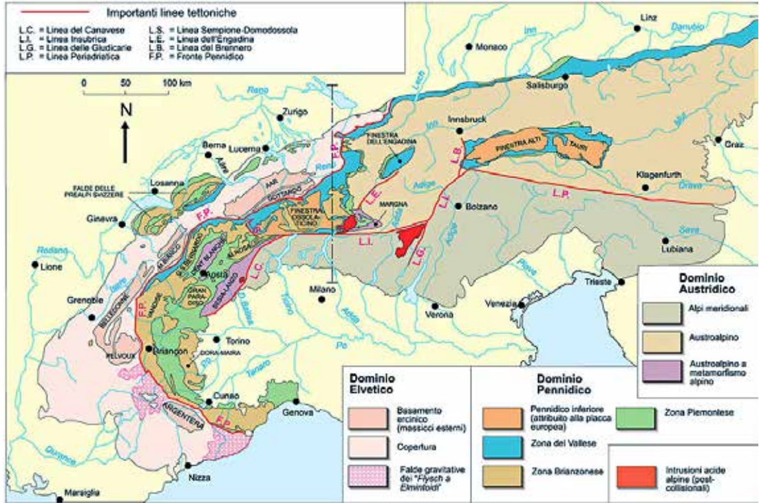
[Figura 283] - Schema tettonico delle Alpi. In questa cartina si vede molto bene la faglia Brianzese. L'autore ha attribuito al Brianzese i massicci cristallini interni (Gran Paradiso, Dora-Maira e Monte Rosa). Quello che qui l'autore indica con piemontese è il pennidico superiore riconducibile all' Oceano Ligure-Piemontese, mentre le Alpi Meridionali sono il sudalpino – da Wikipedia
